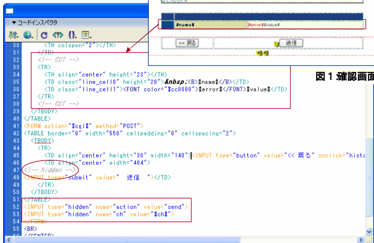
図2 HTMLソース
